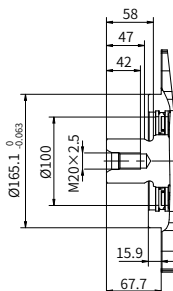
“E6” 型花键轴
