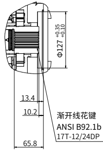
“CG”型通轴驱动
